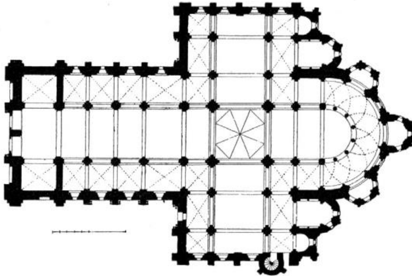
Plan de l'abbatiale de Sainte Foy à Conques
